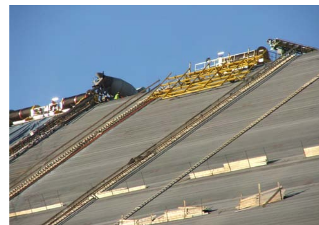
Attrezzature per getto paramento diga
